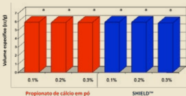
Figura 3- Efeito dos conservantes no volume específico dos pães após forneamento (colunas com letras distintas diferem significativamente entre si; p < 0,05 )
